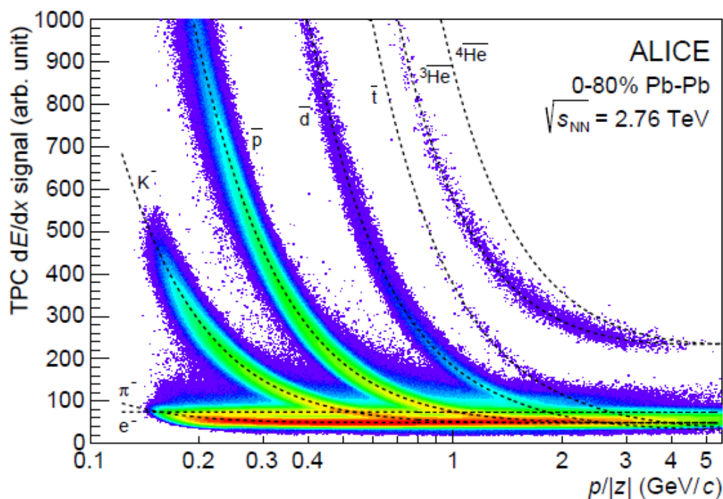
Рис.2 . Идентификация античастиц с помощью временипроекционной камеры (TPC) детектора ALICE.
