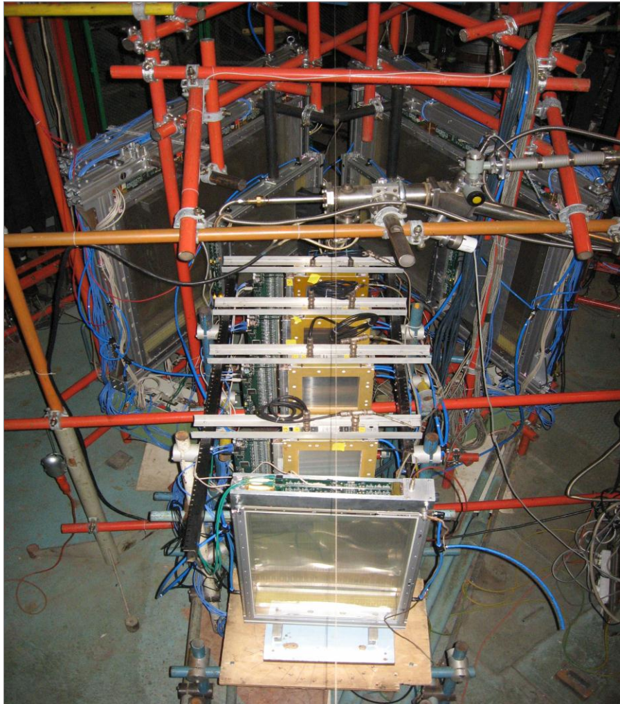
Figure 1. Device «EPECUR»
