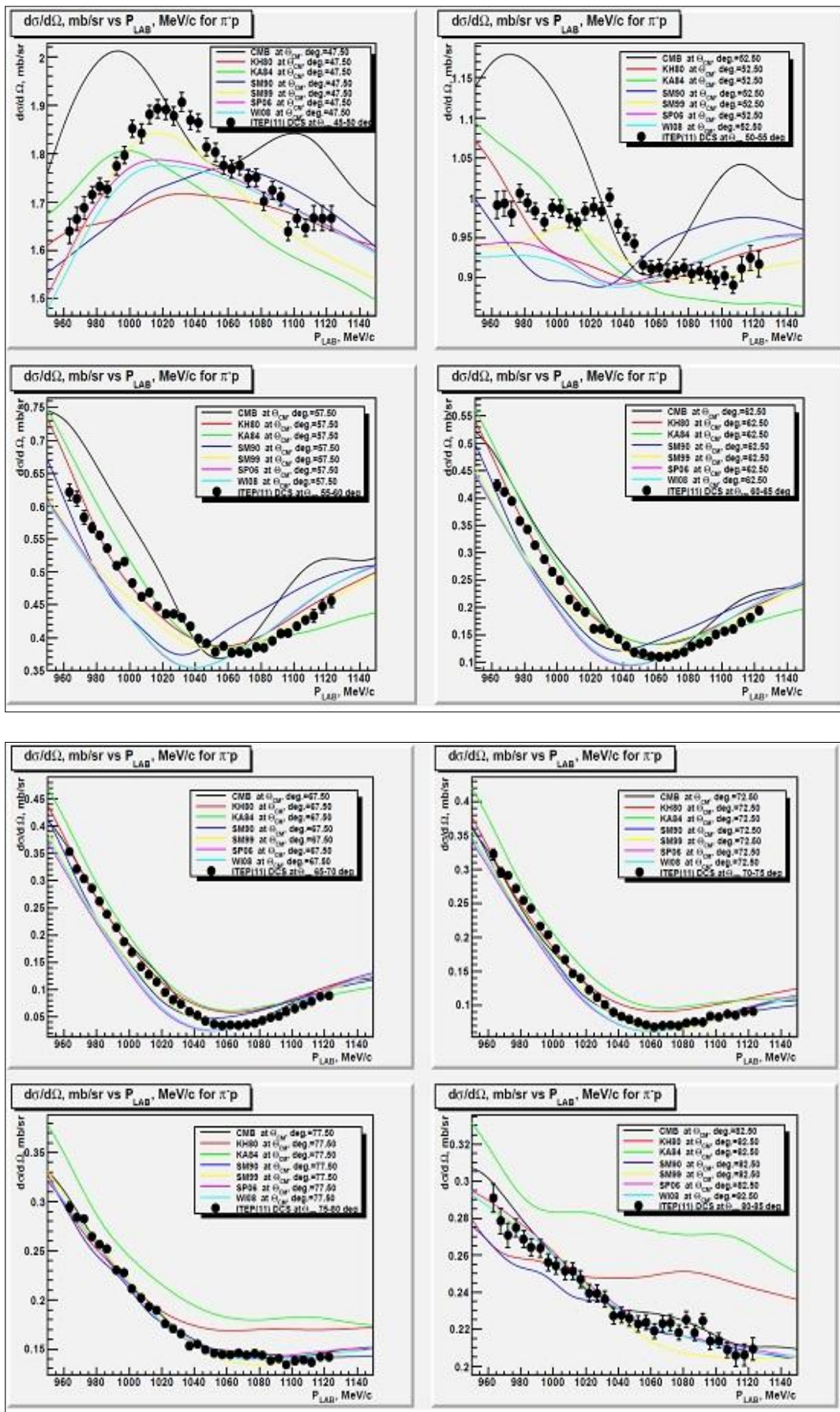
Рис. 3. Дифференциальное сечение упругого рассеяния отрицательных пионов на протонах как функция импульса налетающего пучка в интервалах углов 5 град. (Предварительно).
