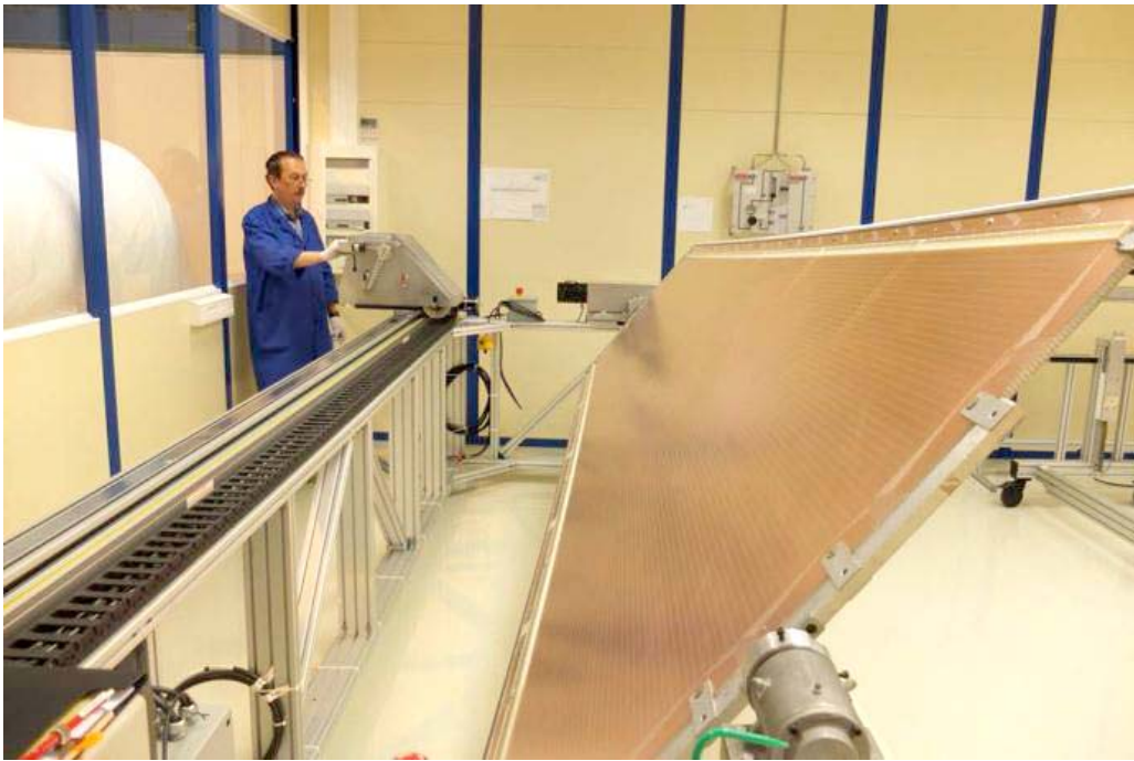
Намотка провололочек на анодную панель
