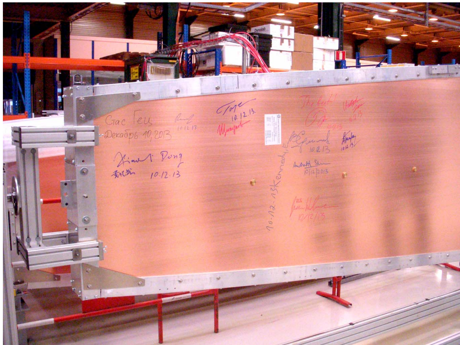
Последняя собранная и оттестированная камера
