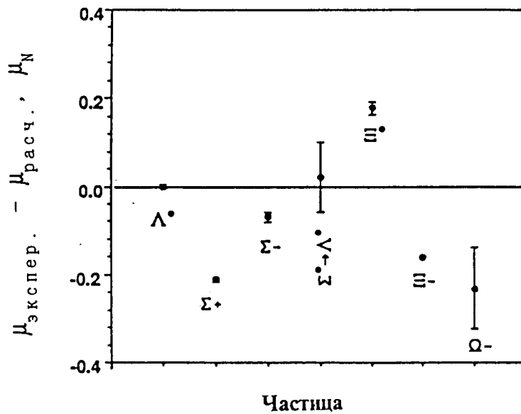
Рис.7. Сравнение экспериментальных значений магнитных моментов с вычисленными в рамках составной кварковой модели.
